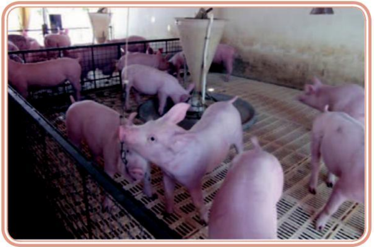
Figura 4.6: Creche com gaiolas de piso vazado
